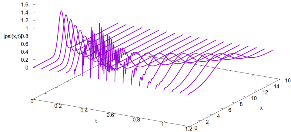
Figure 3: Leapfrog bậc 4 với \sigma_0 = 0.5 và k_0 = -10 : bó sóng truyền về phía -x , phản xạ ở biên trái rồi đổi chiều.
