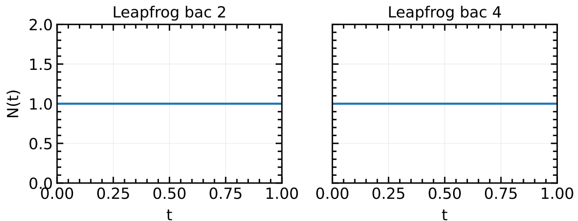
Figure 2: Chuẩn xác suất N(t) của Leapfrog bậc 2 và bậc 4. Hai ô dùng chung giới hạn trục tung.
